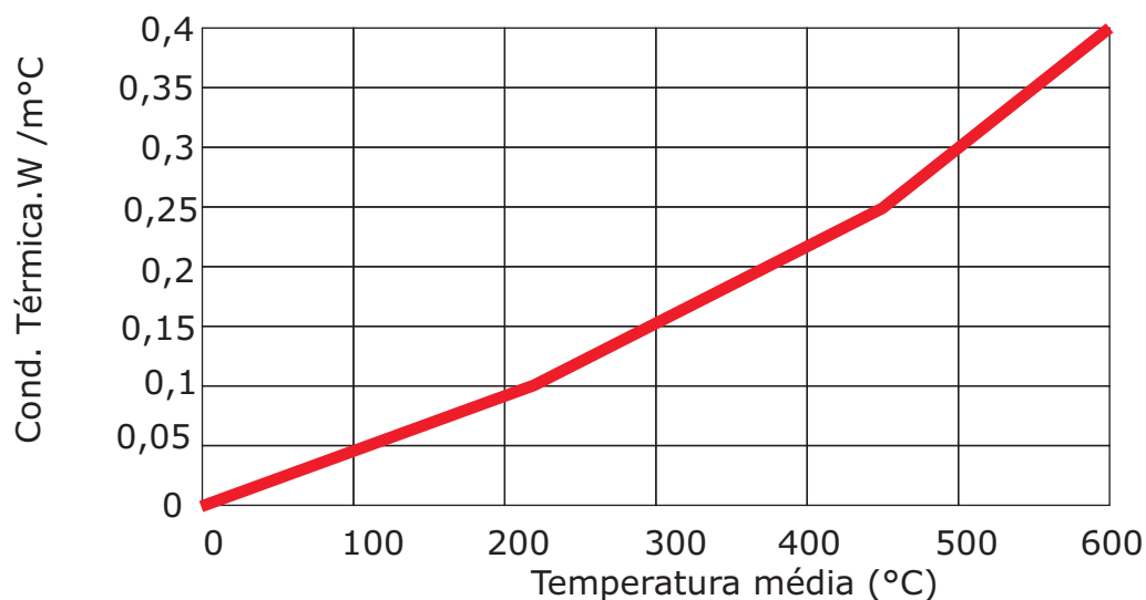
Teste de condutividade térmica x temperatura média
