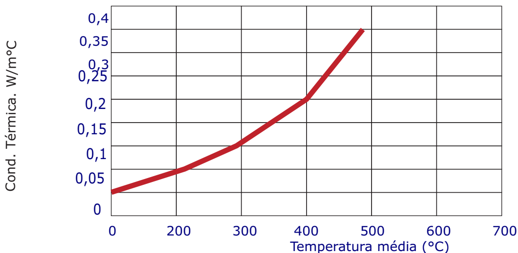
Teste de condutividade térmica x temperatura média
